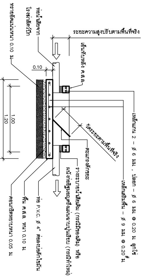
รูปตัดตะกอนดักขยะ 1 : 25
